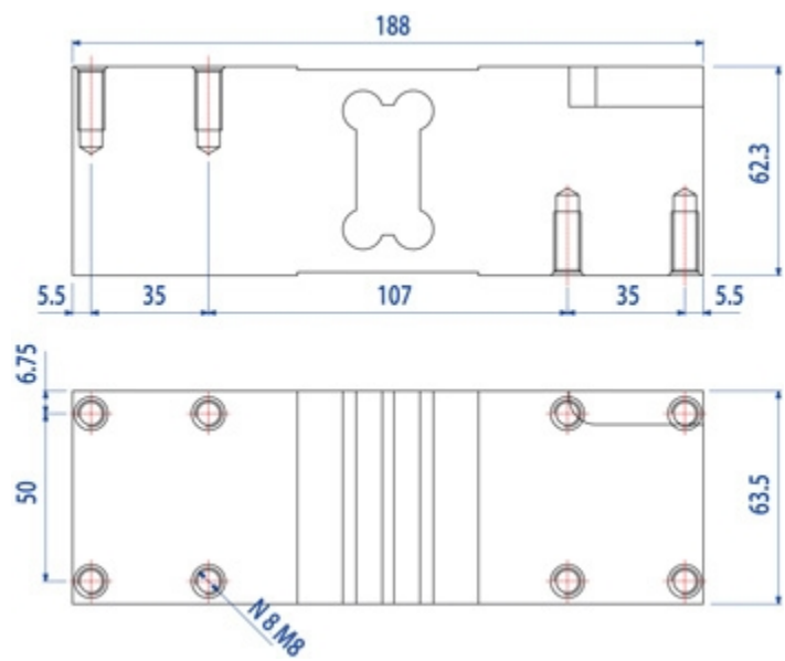
Dimensioni (mm)
